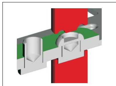
Bild zeigt: Vernieten
